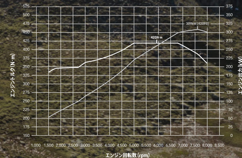
718スパイダー: 309kW(420PS) / 7,600rpm、420N・m/5,000-6,800rpm
