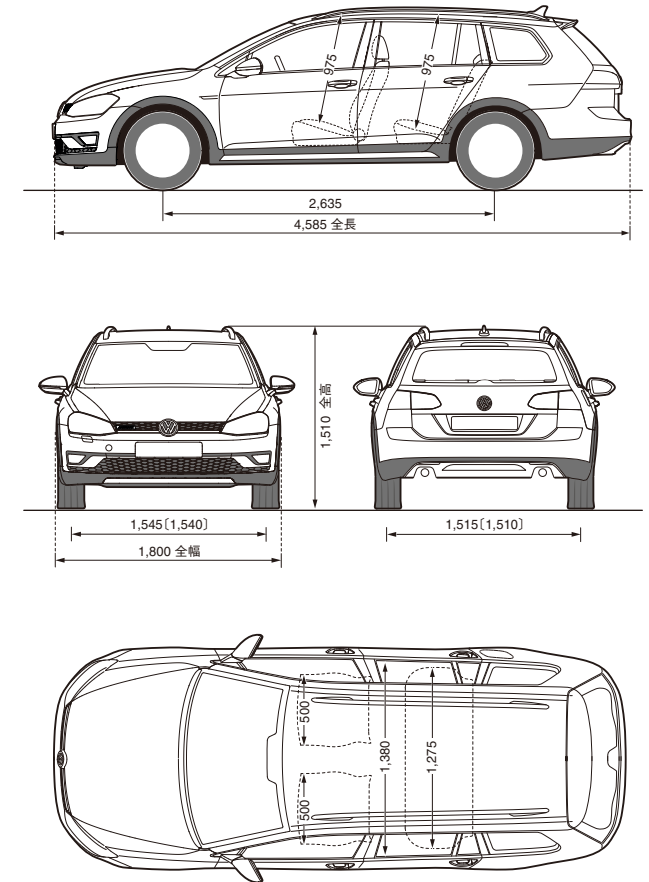
四面図(mm)
